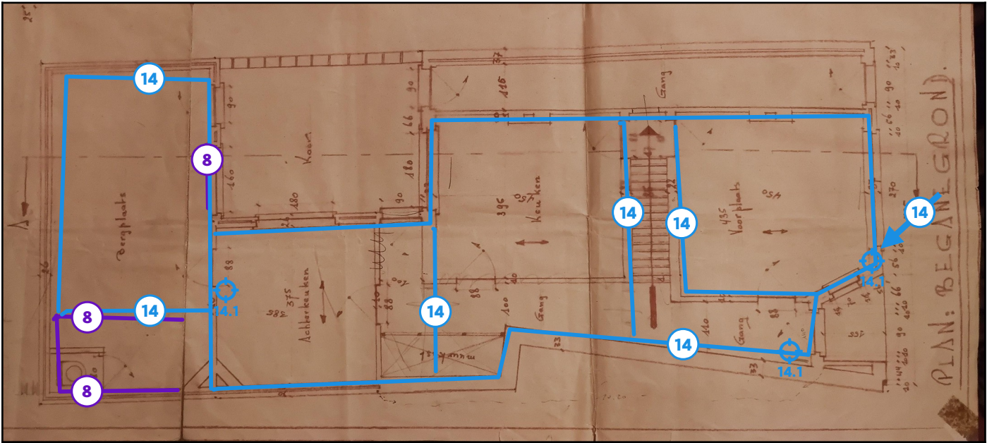
Legende van plan 1.3: gelijkvloers wanden
